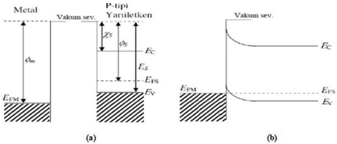
Şekil 3.2. \Phi_m > \Phi_s durumu için metal/p-tipi yarıiletken kontakta enerji-bant diyagramı a) kontakta önce b) kontakta sonra ısısal denge
