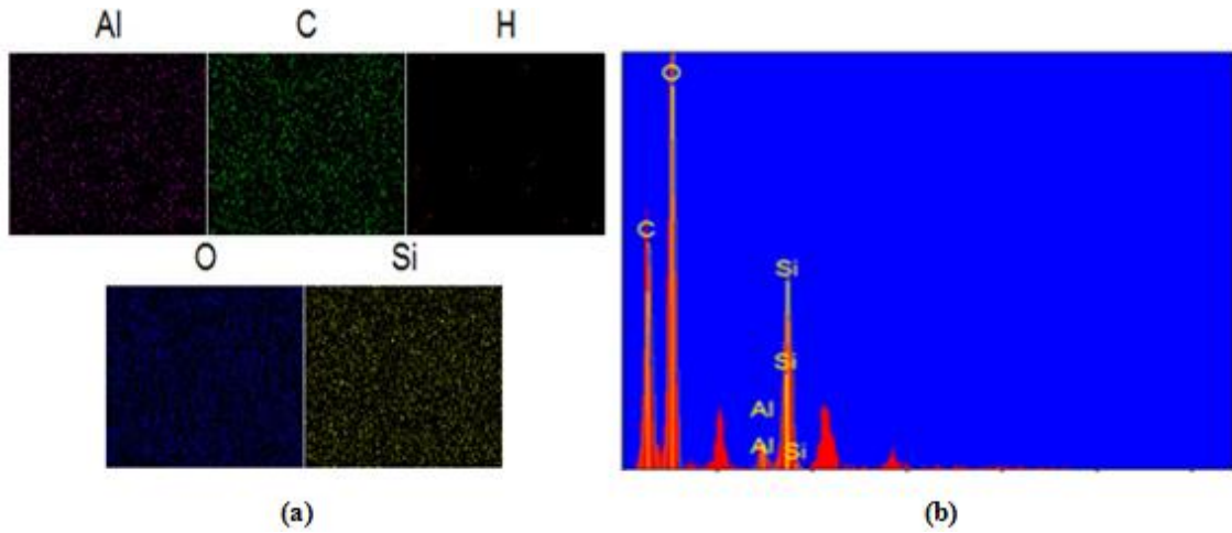
Şekil 5.3. SEM’de görüntülenen elementlerin a) yüzeyssel dağılımları ve b) yoğunluk oranları
