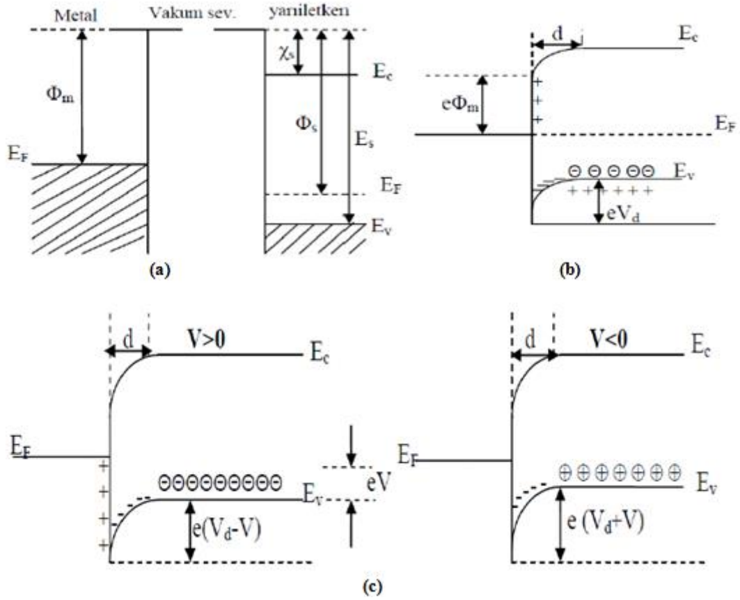
Şekil 3.1. Metal p-tipi Yarıiletken Doğrultucu Konağın Enerji Bant Diyagramı a) Kontakdan önce b) Kontakdan sonra c) V > 0 durumunda ve V < 0 durumunda
