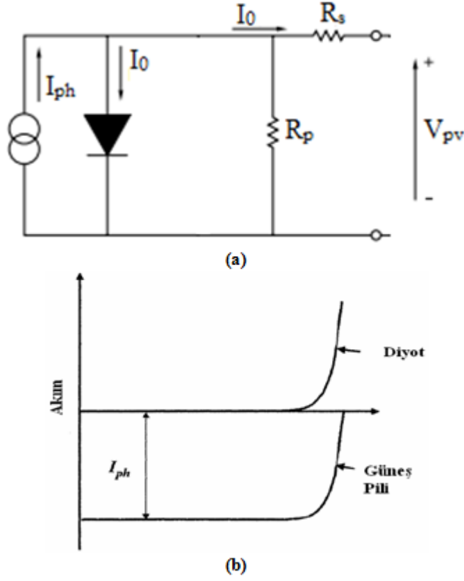
Şekil 3.5. a) Güneş piline ait eşdeğer devrenin gösterimi b) diyot ve güneş piline ait akım-gerilim grafiği
