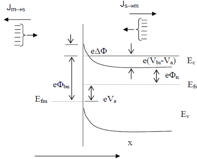
Şekil 3.4. Düz beslem altındaki metal yarıiletken Schottky kontaktaki imaj azalma etkisine ait enerji–band diyagramı
