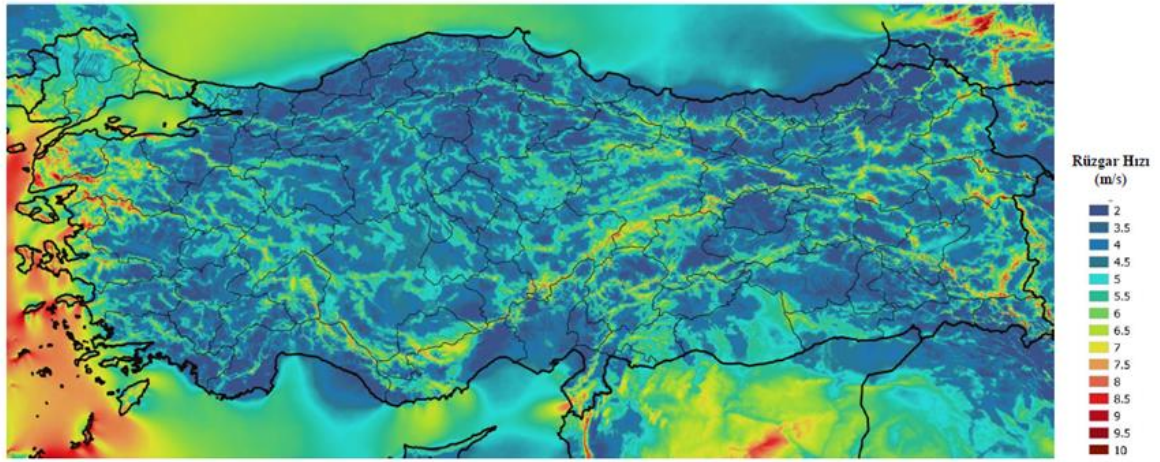
Şekil 3.4. Yıllık ortalama rüzgâr hızı dağılımı-100m [37]
