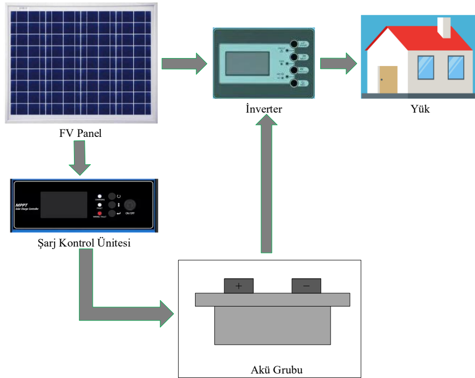
Şekil 3.10. Şebekeden bağımsız bir FV sistemin genel yapısı
