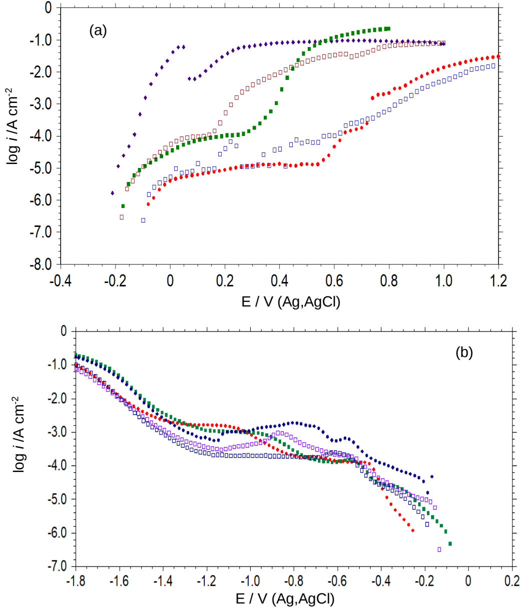
Şekil 4.2. Cu elektrodun farklı derişimlerde (10: ●, 5: ○, 1: ■, 0,5: ◆, 0,1: □) Rh içeren %3,5 NaCl çözeltilerde elde edilen anodik (a) ve katodik (b) yarı logaritmik akım – potansiyel eğrileri
