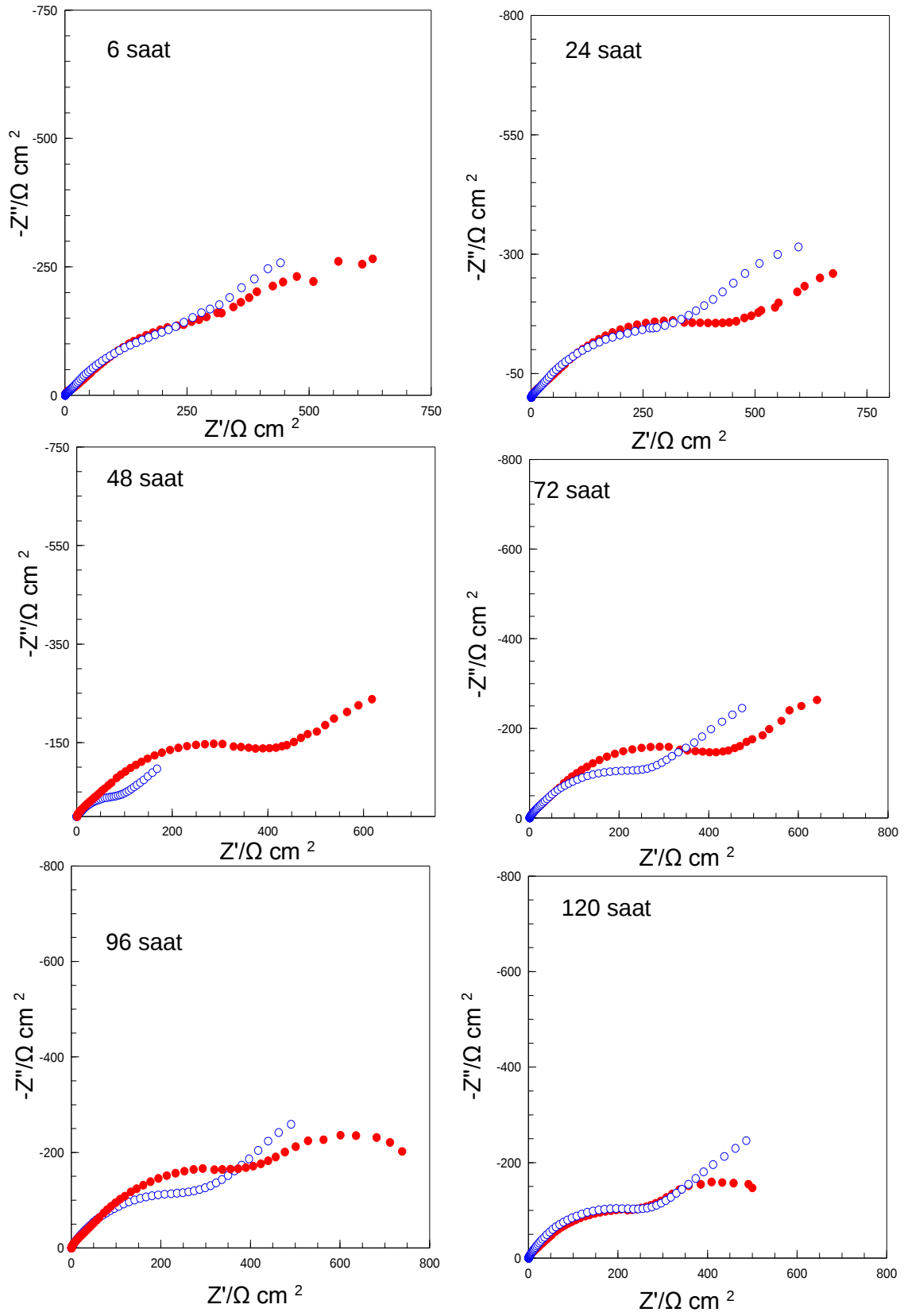
Şekil 4.9. Cu'nın 10 Mm Rh içeren (●) ve içermeyen (○) %3,5 NaCl çözeltisinde farklı zamanlarda (6 s – 120 saat) elde edilen Nyquist eğrileri
