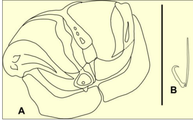
Şekil 3.3. P. bingolensis ; A:Kanca yapısı (Skala; 100 µm); B Orta kanca (Civáňová et al. 2013)
