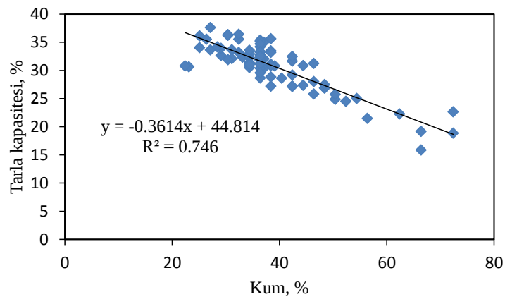
Şekil 4.1. Toprak kum içeriği ile tarla kapasitesi ilişkisi
