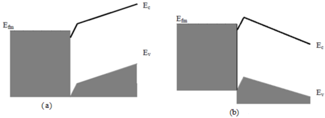
Şekil 3.4. ( \Phi_m < \Phi_s ) durumu için metal/n-tipi yarıiletken omik kontakta ait enerji bant diyagramı a) Ters beslem altında, b) Düz beslem altında
