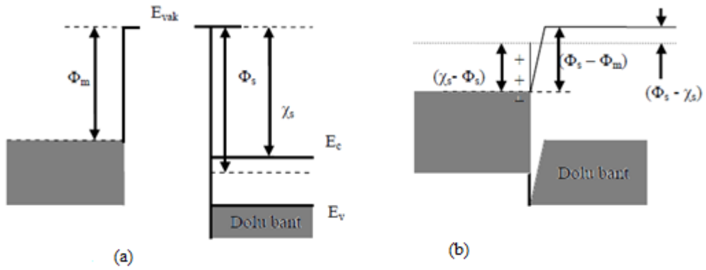
Şekil 3.3. ( \Phi_m < \Phi_s ) durumu için metal/n-tipi yarıiletken omik kontakta ait enerji bant diyagramı a) Kontakтан önce, b) Kontakтан sonra
