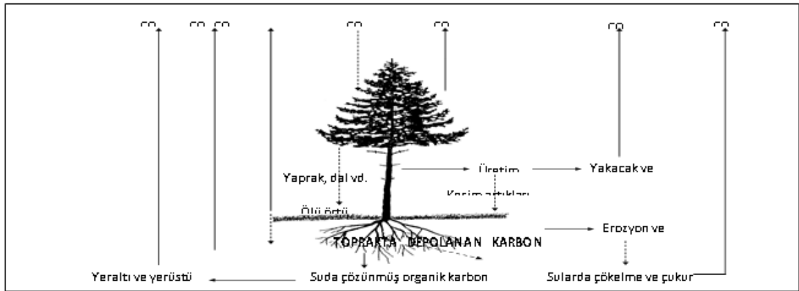
Şekil 2.2. Orman ekosistemlerinde karbon döngüsü (Lal 2004) (düz çizgiler karbon çıkışını, kesik çizgiler karbon girdisini göstermektedir)
