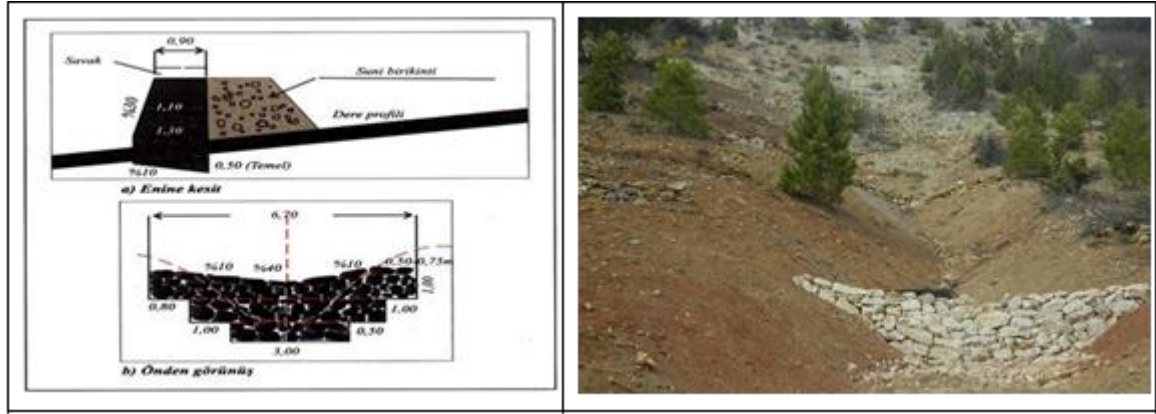
Şekil 4.15. Kuru duvar eşik şekli ve örnek kuru duvar (ÇEM Arşiv)
