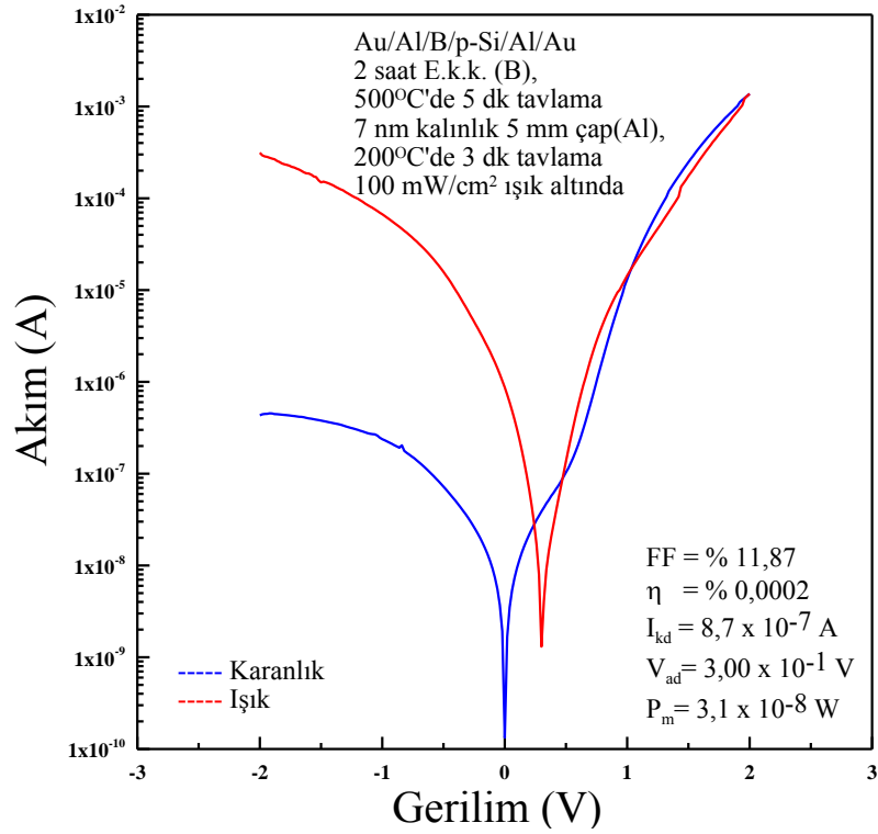
Şekil 4.10. Au/Al/p-Si/B/Al/Au yapısının 200°C'de 3 dk tavlama ile elde edilen yarı logaritmik Akım-Gerilim grafiği
