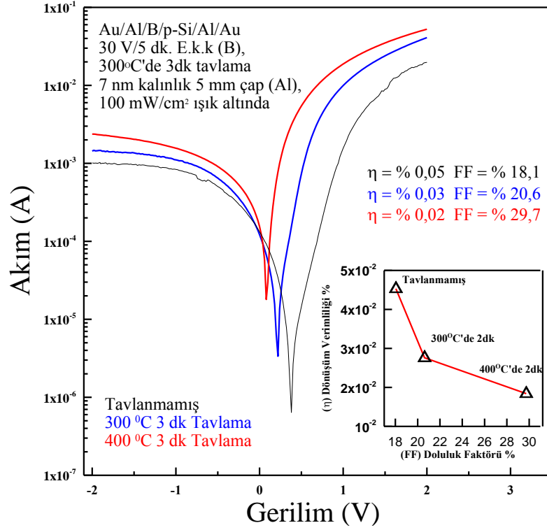
Şekil 4.15. Au/Al/B/p-Si/Al/Au yapısının farklı sıcaklıklara bağlı tavlama değerleri için yarı logaritmik Akım-Gerilim Grafiği. Küçük grafikte tavlama değerleri olarak Değişen FF ve η değerlerinin değişimi
