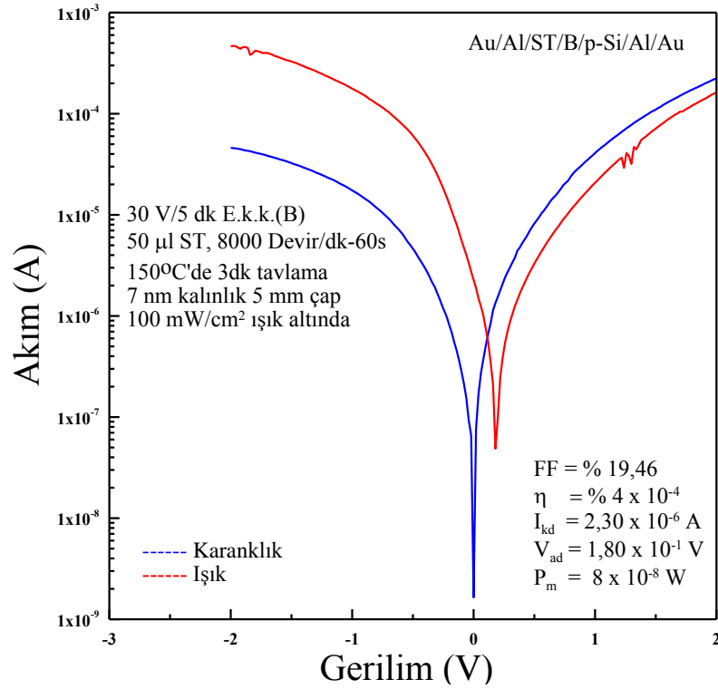
Şekil 4.16. Au/Al/ST/B/p-Si/Al/Au yapısının 150°C 3dk tavlama değerleri için yarı logaritmik Akım-Gerilim grafiği
