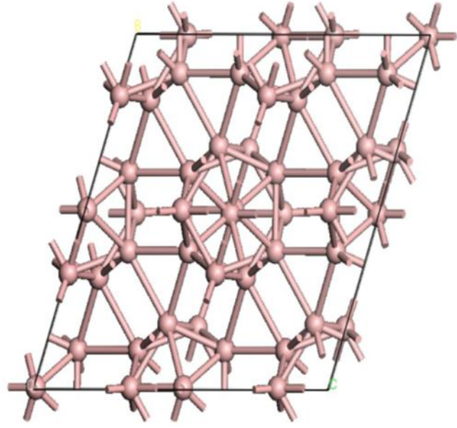
Şekil 3.1. Bor'un kristal yapısı (Xiaoju et al. 2006)
