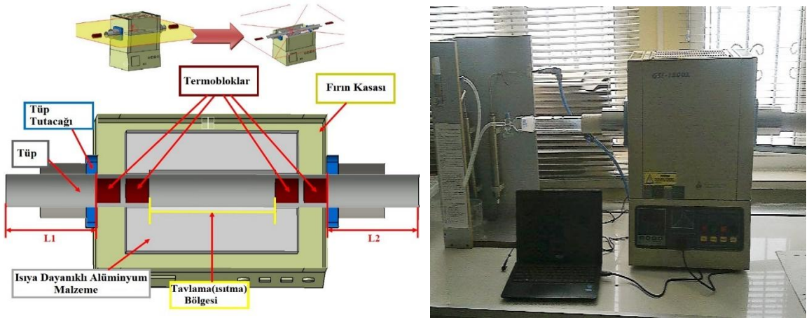
Şekil 3.15. Tavlama fırını şematik (Url 4'ten uyarlandı) ve resim ile gösterimi
