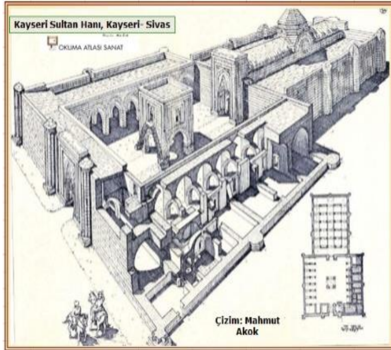
Görseller 3.2.7.1: Tuzluhisar Sultan Hanı Planı ( http://sanatokuma.blogspot.com/p/anadolu-selcuklu-mimarisi-iii.html Erişim Tarihi: 29.01.2022.)
