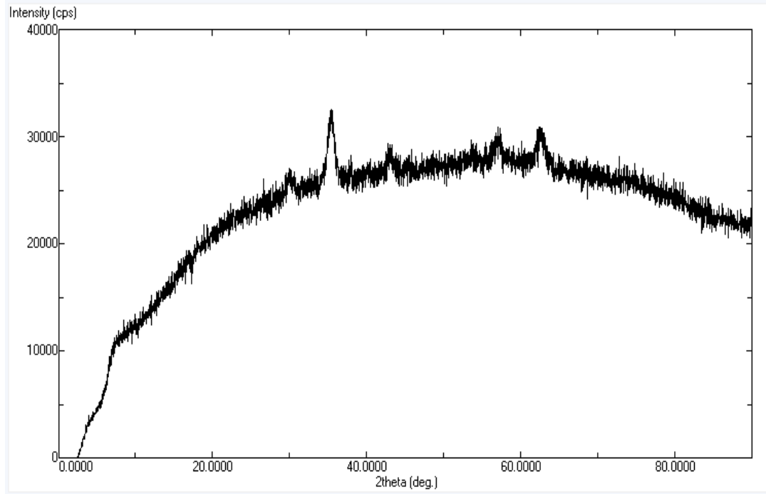
Şekil 4.2. Yeşil sentez metodu ile sentezlenen FeNP1'nin XRD grafiği
