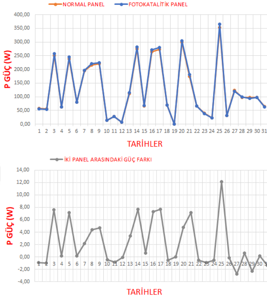
Şekil 6.5. Ocak Ayı Güç Grafikleri
