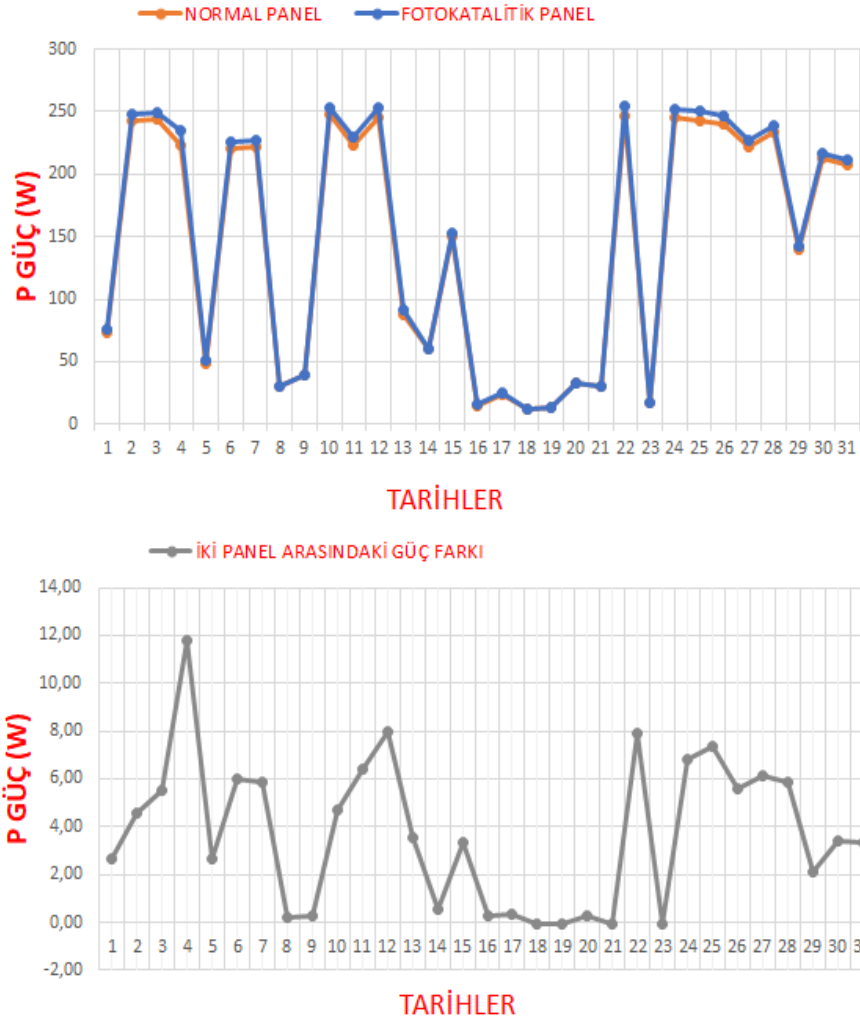
Şekil 6.4.. Aralık Ayı Güç Grafikleri
