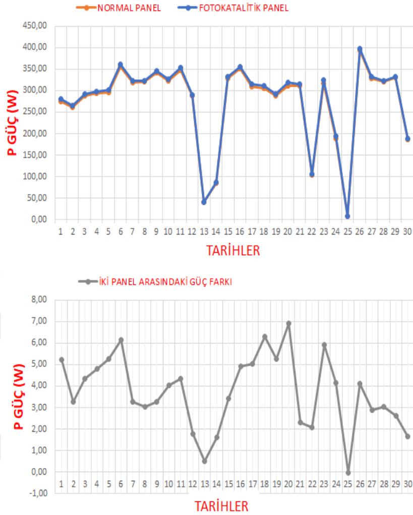
Şekil 6.10. Haziran Ayı Güç Grafikleri
