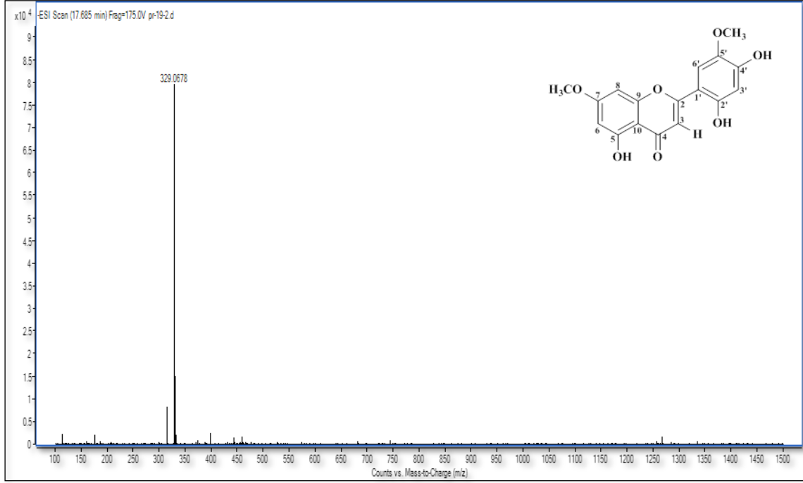
Şekil 4.17. 7,5'-dimetoksiisoeugenin (1) bileşięininin HRESIMS kromatogramı
