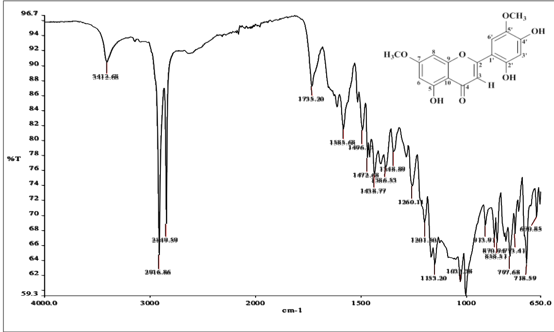
Şekil 4.16. 7,5'-dimetoksiizoeitin (1) bileşiğinin FT-IR spektrumu
