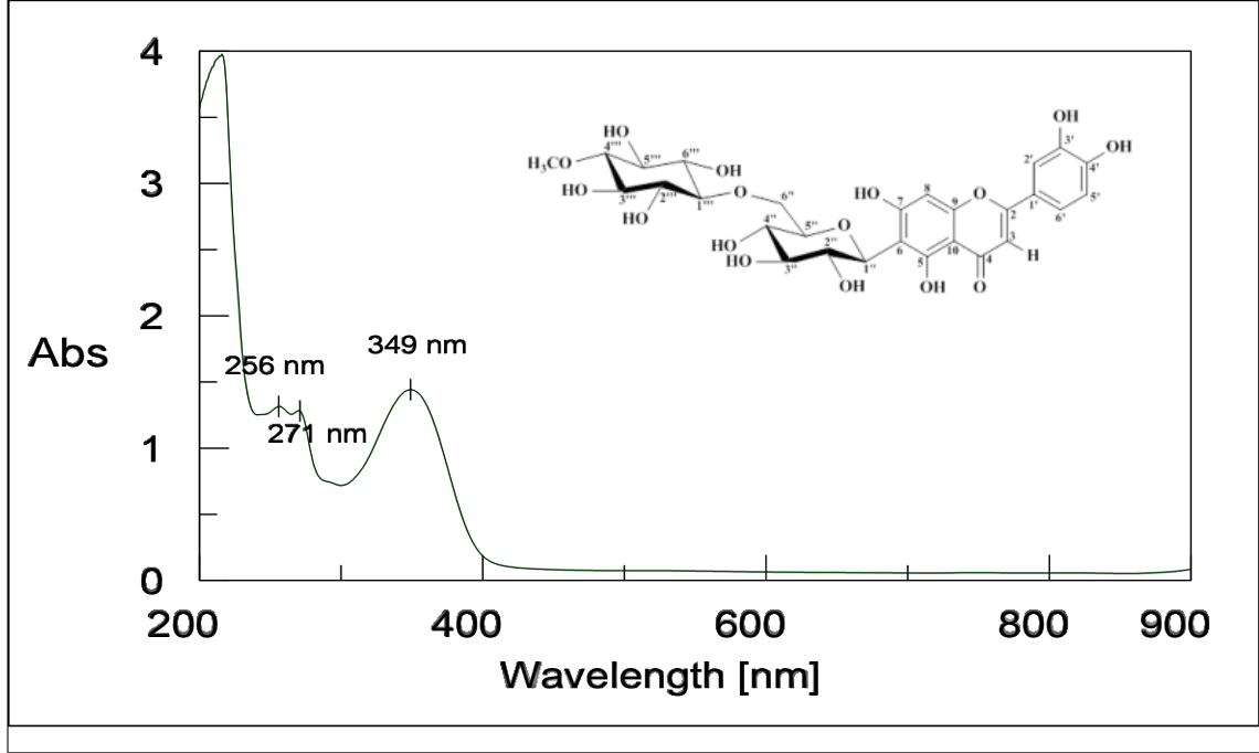
Şekil 4.36. Homoorientin-6''-4- O -metil- myo -inositol (2) bileşiğinin UV-VIS spektrumu
