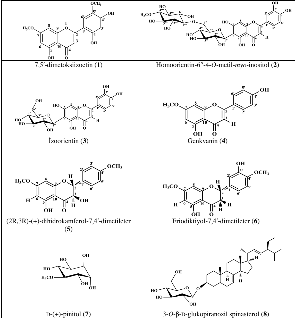
Şekil 4.6. P. ortegoides türünden izole edilen bileşiklerin kimyasal yapıları
