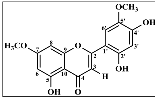
Şekil 4.8. 7,5'-dimetoksiizoetin (1) bileşiğinin kimyasal yapısı
