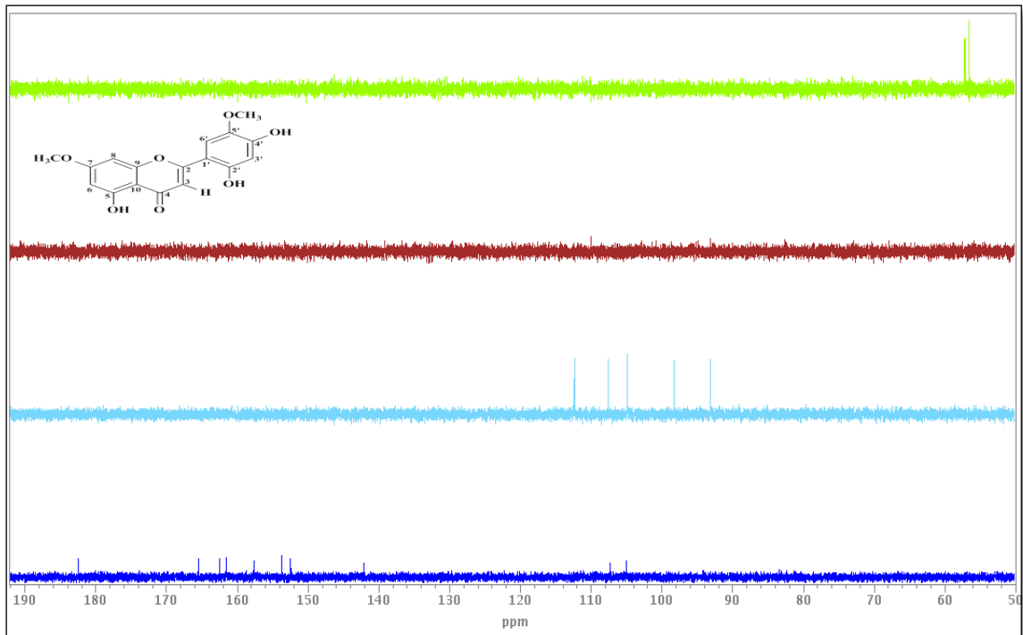
Şekil 4.11. 7,5'-dimetoksiisoeugenin (1) bileşiğinin ^{13}\text{C} -DEPT NMR spektrumu ( ^{13}\text{C} : 125 MHz; \text{DMSO-}d_6 )
