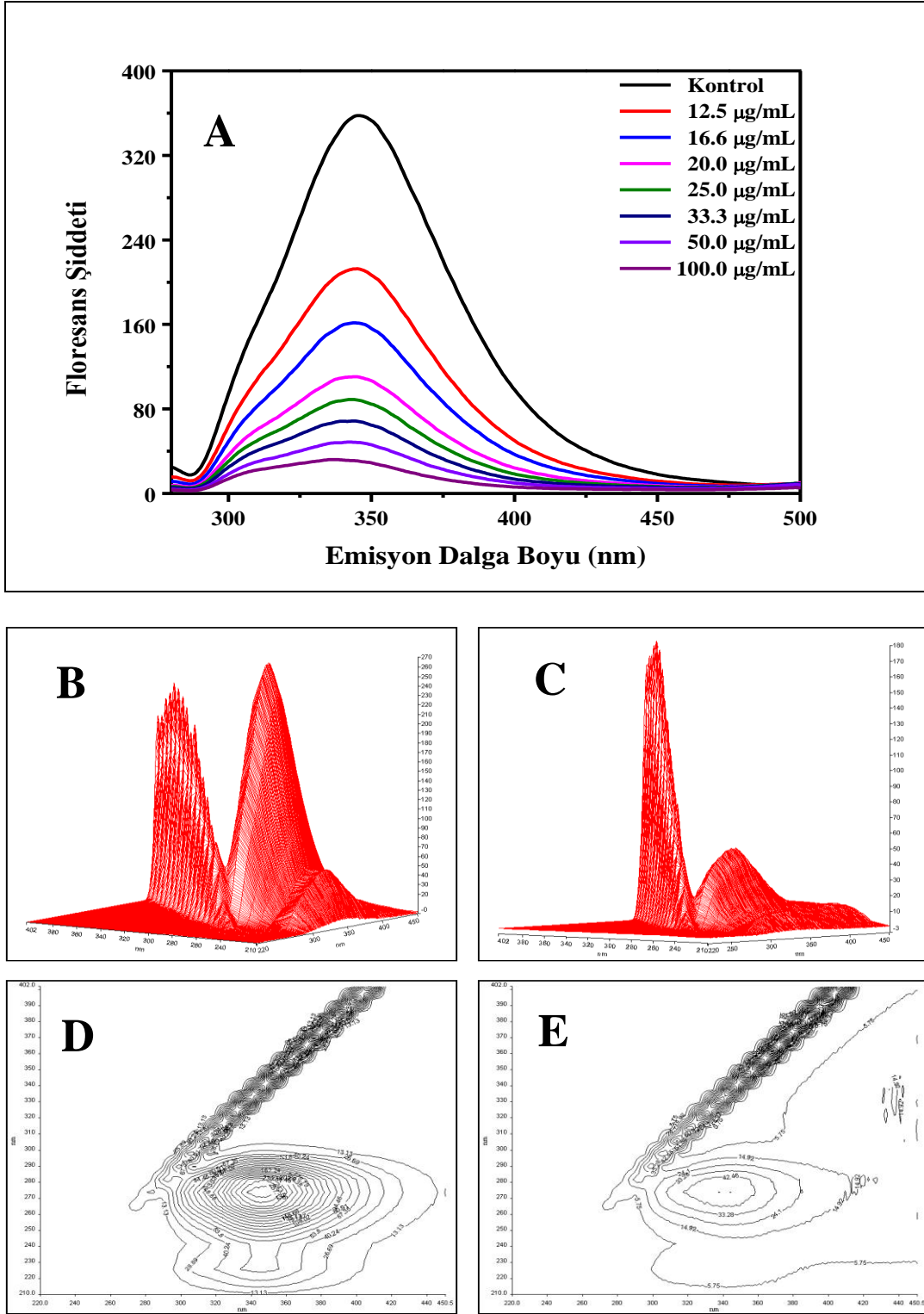
Şekil 4.55. (A) Farklı konsantrasyonlardaki 7,5'-dimetoksiisoeugenol (1) molekülünün HSA proteini ile etkileşiminden elde edilen 2D-FL spektrumları. (B) HSA proteininin 3D-FL spektrumu ( 5 \times 10^{-6} M). (C) HSA ( 5 \times 10^{-6} M) + 7,5'-dimetoksiisoeugenol (1) sisteminin (50 µg/mL) 3D-FL spektrumu. (D) HSA proteininin 3D harita yüzey spektrumu ( 5 \times 10^{-6} M). (E) HSA ( 5 \times 10^{-6} M) + 7,5'-dimetoksiisoeugenol (1) sisteminin (50 µg/mL) 3D harita yüzey spektrumu. 3D-FL spektrumlarında x eksenini emisyon dalga boyu ( \lambda_{em} ), y eksenini uyarma dalga boyu ( \lambda_{ex} ) z eksenini ise floresans şiddetini göstermektedir. 3D harita yüzey spektrumlarında x eksenini emisyon dalga boyunu ( \lambda_{em} ), y eksenini uyarma dalga boyunu ( \lambda_{ex} ) göstermektedir
