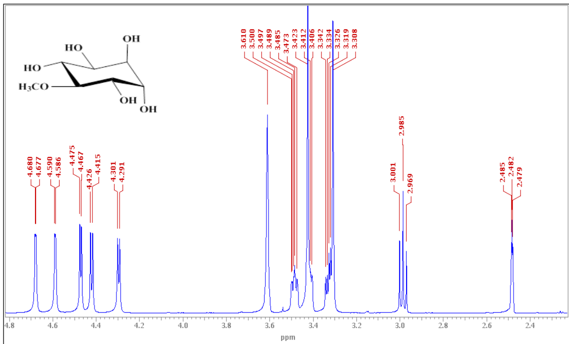
Şekil 4.50. D-(+)-pinitol (7) bileşiğinin 1 H-NMR spektrumu ( 1 H: 600 MHz; DMSO- d 6 )
