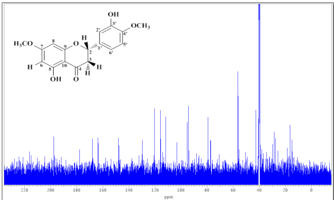
Şekil 4.48. Eriodiktıyol-7,4'-dimetileter (6) bileşiğinin 13 C-NMR spektrumu ( 13 C: 125 MHz; DMSO- d 6 )
