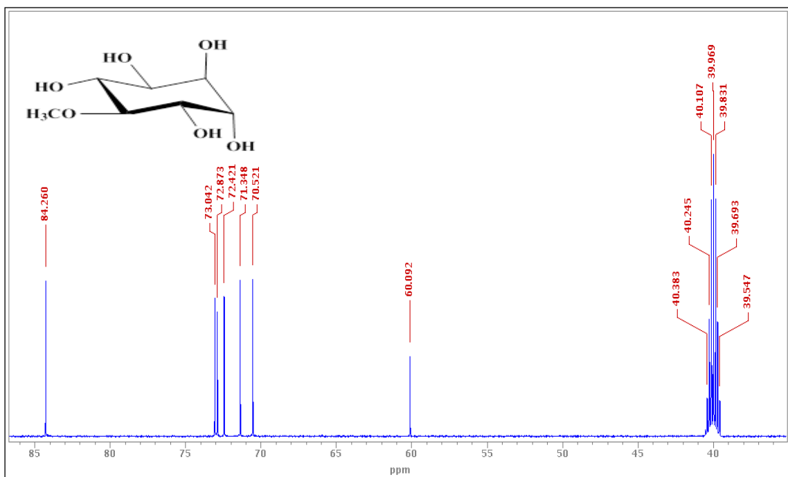
Şekil 4.51. D-(+)-pinitol (7) bileşiğinin 13 C-NMR spektrumu ( 13 C: 125 MHz; DMSO- d 6 )
