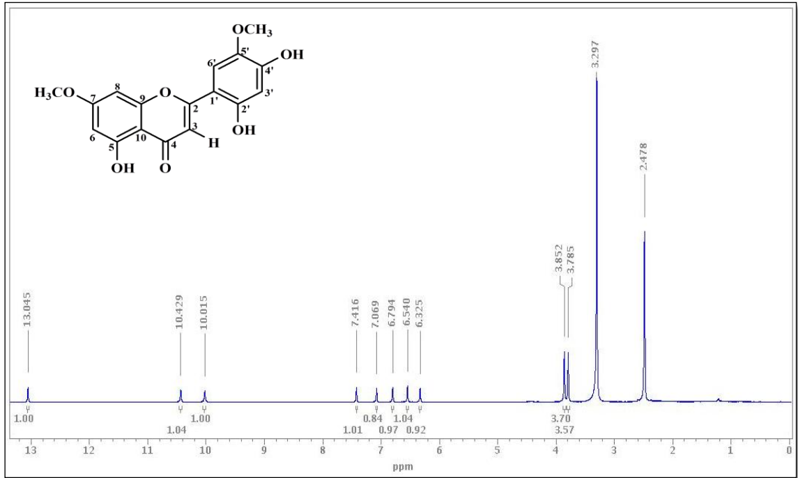
Şekil 4.9. 7,5'-dimetoksiizoeatin ( ^1\text{H} -NMR spektrumu ( ^1\text{H} : 600 MHz; \text{DMSO}-d_6 )
