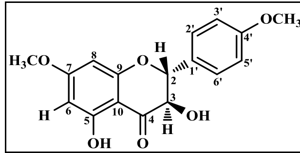
Şekil 4.43. (2R,3R)-(+)-dihidrokamferol-7,4'-dimetileter (5) bileşiđinin kimyasal yapısı
