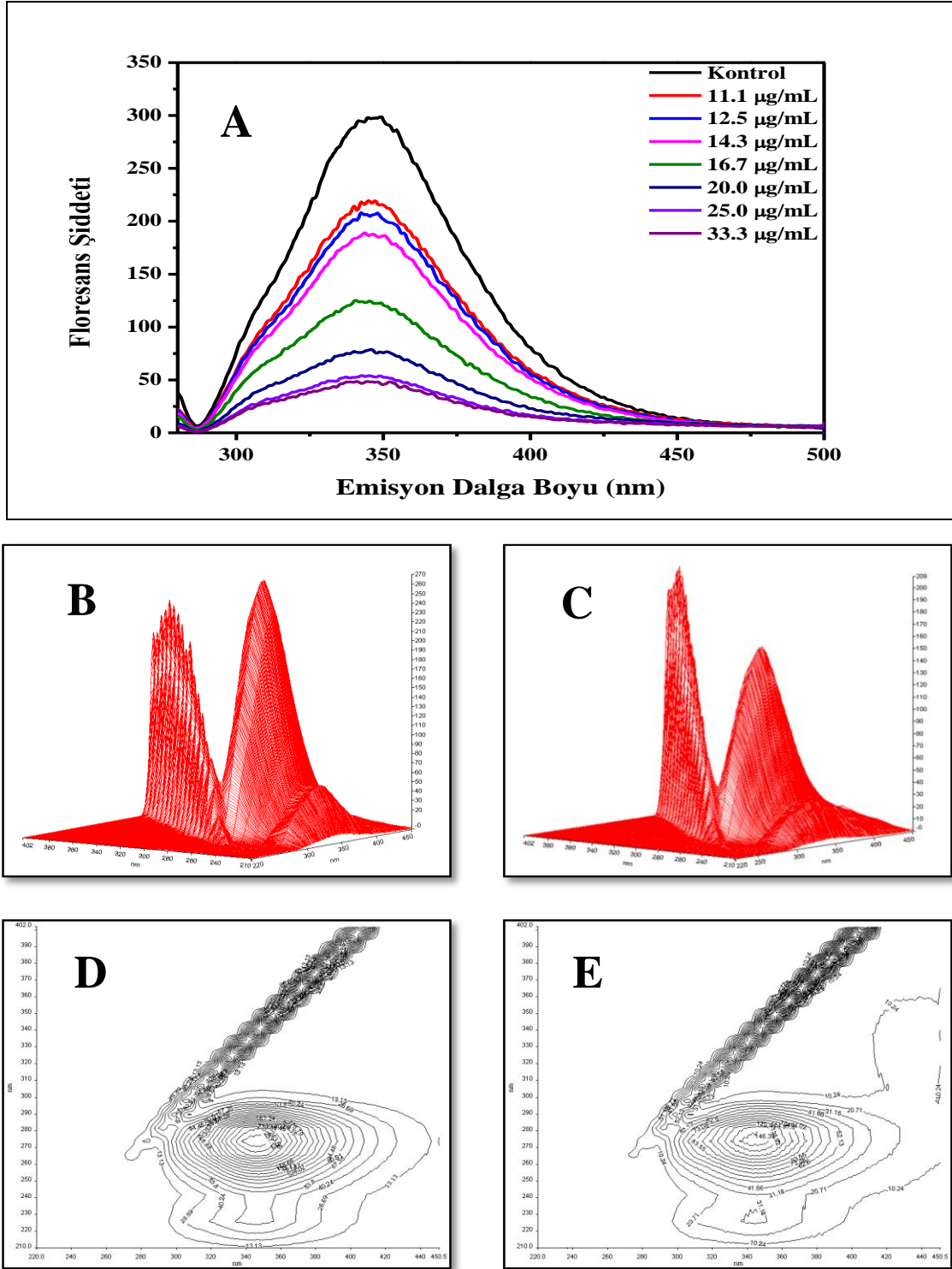
Şekil 4.59. (A) Farklı konsantrasyonlardaki (2R,3R)-(+)-dihidrokamferol-7,4'-dimetileter molekülünün HSA proteini ile etkileşiminden elde edilen 2D-FL spektrumları. (B) HSA proteininin 3D-FL spektrumu ( 5 \times 10^{-6} M). (C) HSA ( 5 \times 10^{-6} M) + (2R,3R)-(+)-dihidrokamferol-7,4'-dimetileter sisteminin (50 µg/mL) 3D-FL spektrumu. (D) HSA proteininin 3D harita yüzey spektrumu ( 5 \times 10^{-6} M). (E) HSA ( 5 \times 10^{-6} M) + (2R,3R)-(+)-dihidrokamferol-7,4'-dimetileter sisteminin (50 µg/mL) 3D harita yüzey spektrumu. 3D-FL spektrumlarında x eksenini emisyon dalga boyu ( \lambda_{em} ), y eksenini uyarma dalga boyu ( \lambda_{ex} ) z eksenini ise floresans şiddetini göstermektedir. 3D harita yüzey spektrumlarında x eksenini emisyon dalga boyunu ( \lambda_{em} ), y eksenini uyarma dalga boyunu ( \lambda_{ex} ) göstermektedir.
