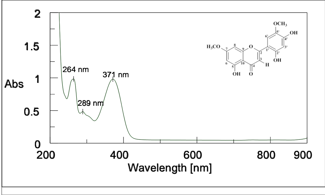
Şekil 4.18. 7,5'-dimetoksiizoeletin (1) bileşiğinin UV-VIS spektrumu
