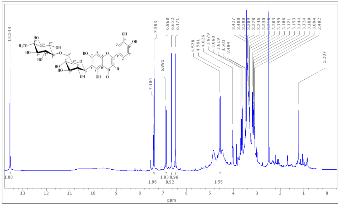
Şekil 4.20. Homoorientin-6''-4-O-metil- myo -inositol (2) bileşiğinin 1 H-NMR spektrumu ( 1 H: 600 MHz; DMSO- d 6 )
