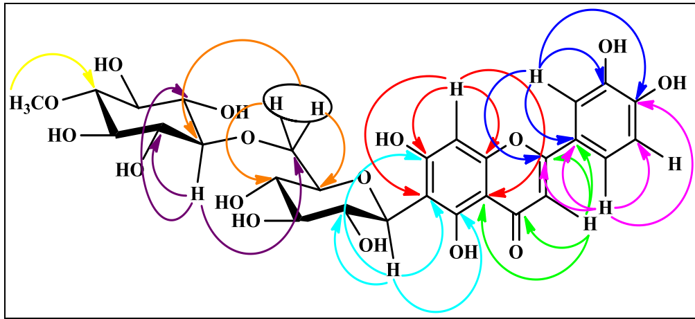
Şekil 4.23. Homoorientin-6''-4-O-metil- myo -inositol (2) bileşiğinin HMBC korelasyonları
