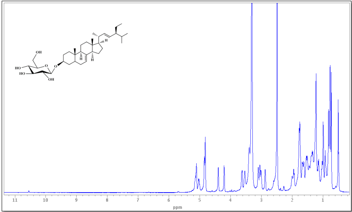
Şekil 4.53. 3- O -β-D-glukopiranozil spinasterol (8) bileşiminin 1 H-NMR spektrumu ( 1 H: 600 MHz; DMSO- d 6 )
