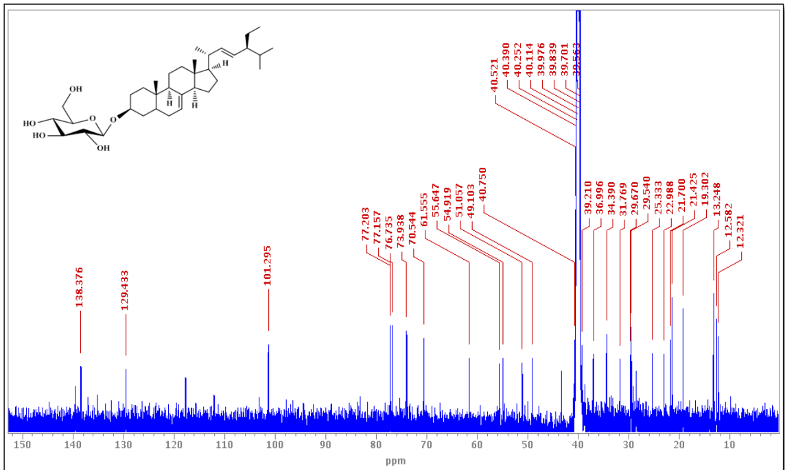
Şekil 4.54. 3- O -β-D-glukopiranozil spinasterol (8) bileşiminin 13 C-NMR spektrumu ( 13 C: 125 MHz; DMSO- d 6 )
