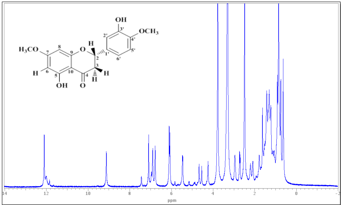
Şekil 4.47. Eriodiktıyol-7,4'-dimetileter (6) bileşiğinin 1 H-NMR spektrumu ( 1 H: 600 MHz; DMSO- d 6 )
